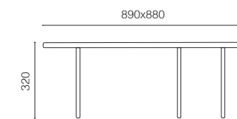
ADA COFFEE TABLE 704
