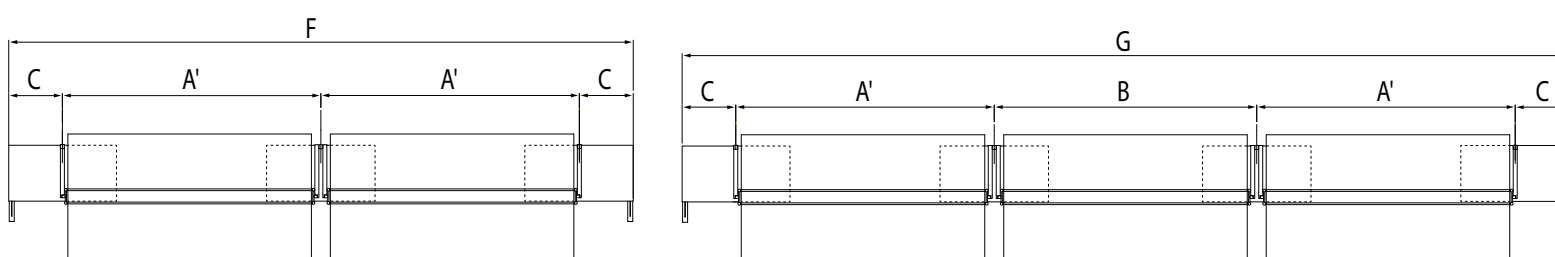
ENTRE-AXES BASE PIASTRA POUR PLUSIEURS FLEXY (MAT CENTRAL DOUBLE)
