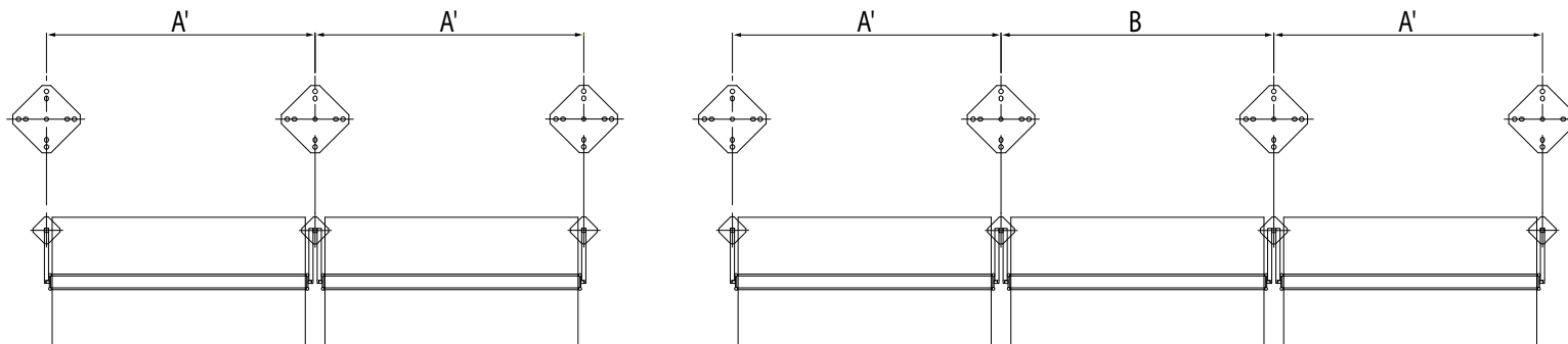
ENTRE-AXES STYLO POUR PLUSIEURS FLEXY (MAT CENTRAL DOUBLE)
