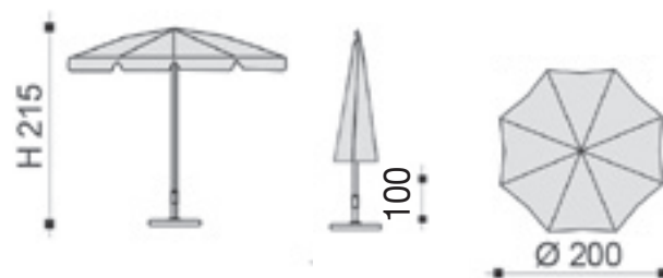
Art. 181A - (palo alluminio/mât alu/alu pole/mastil aluminio)
