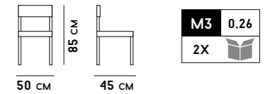
CLAUDE 0181 Sedia cordino con crociera Stacking woven chair
