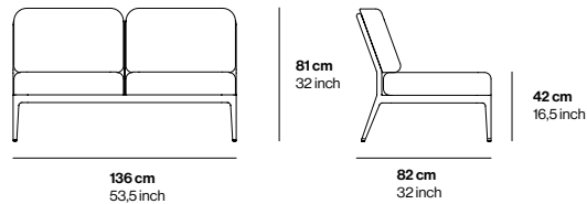
Izquierdo doble Double left
