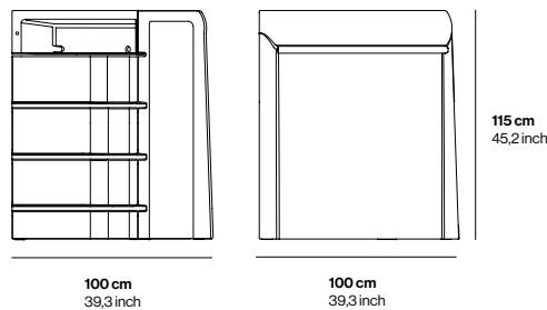
Bar Classe curvo Curved Classe Bar
