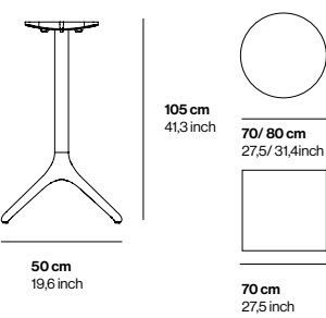
Fijo 105 XL 105 Fixed XL
