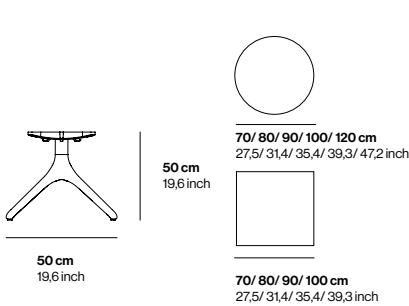
Fijo cerámico 50 XL 50 Ceramic Fixed XL
