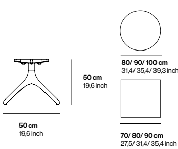
Fijo 50 XL 50 Fixed XL
