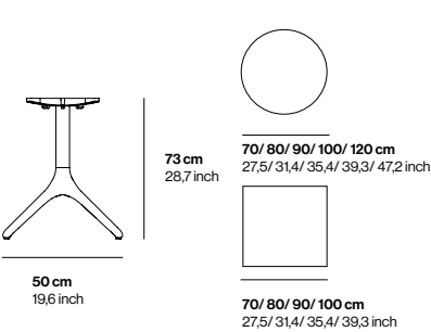
Fijo cerámico 73 XL 73 Ceramic Fixed XL
