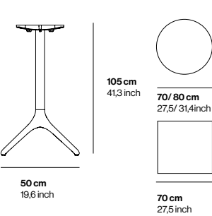
Fijo cerámico 105 XL 105 Ceramic Fixed XL
