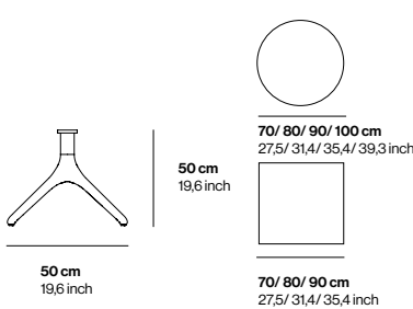
Fijo vidrio 50 XL 50 Glass Fixed XL
