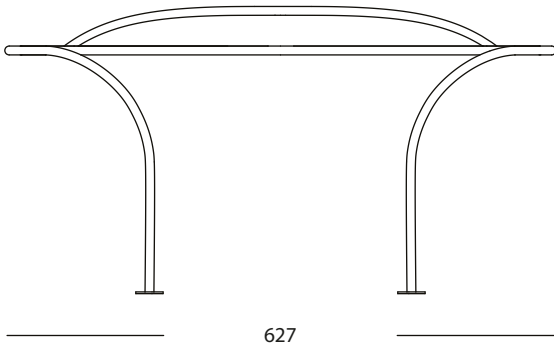
- 76234 Pergola 627 x 385 x h 325 cm
