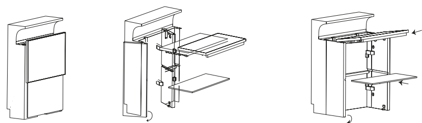
Modulo chiuso Closed element Aprire le due ante e inserire il piano Open the two sides and place the top Inserire la mensola Place the shelf
